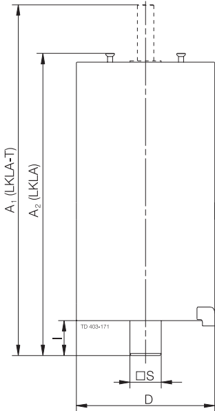
Fig. 2. Dimensions - actuators.
